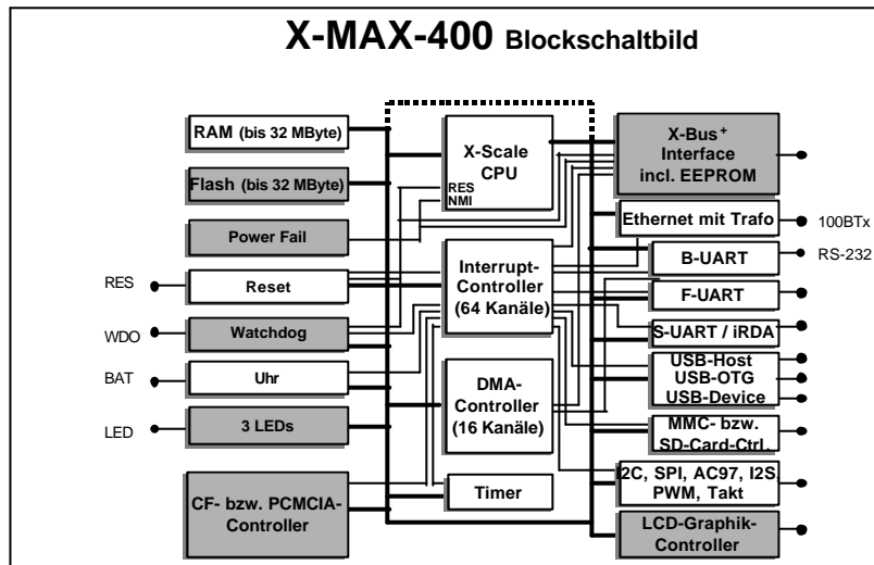
Abb. 2: Blockschaltbild
